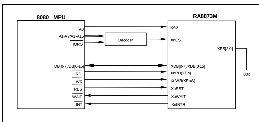
圖 7-1 : 8080 MPU Interface
