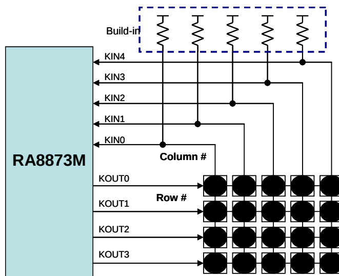
圖 17-1 : Key-Pad Application
