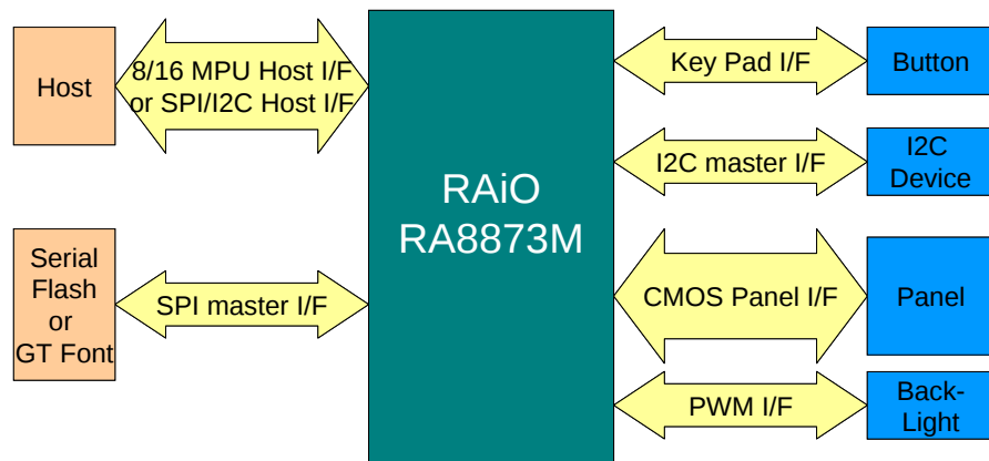
圖 1-1 : System Diagram
