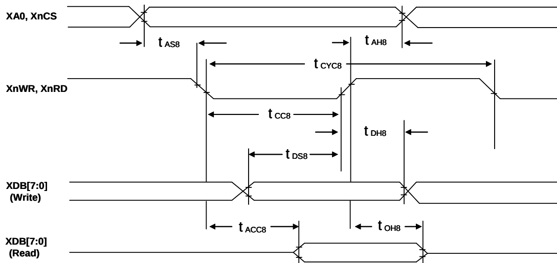
圖 7-3 : 8080 Waveform
