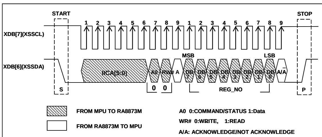
圖 7-22 : CMD Write on IIC-Bus
